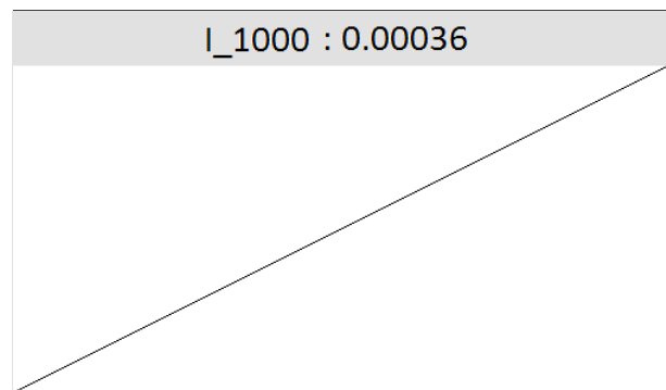
v_n = \sqrt{2} \cdot n \bmod 1 avec n \in [0, 1000]
