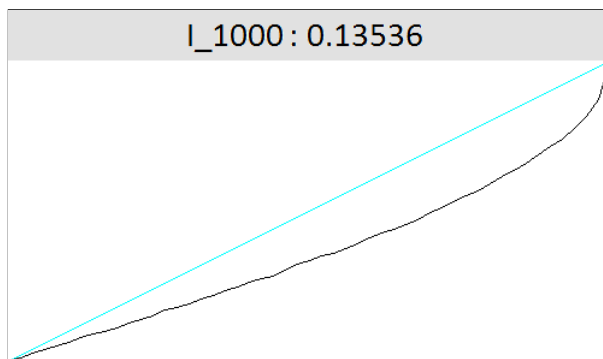
u_n = |\cos(n)| avec n \in [0, 1000]
